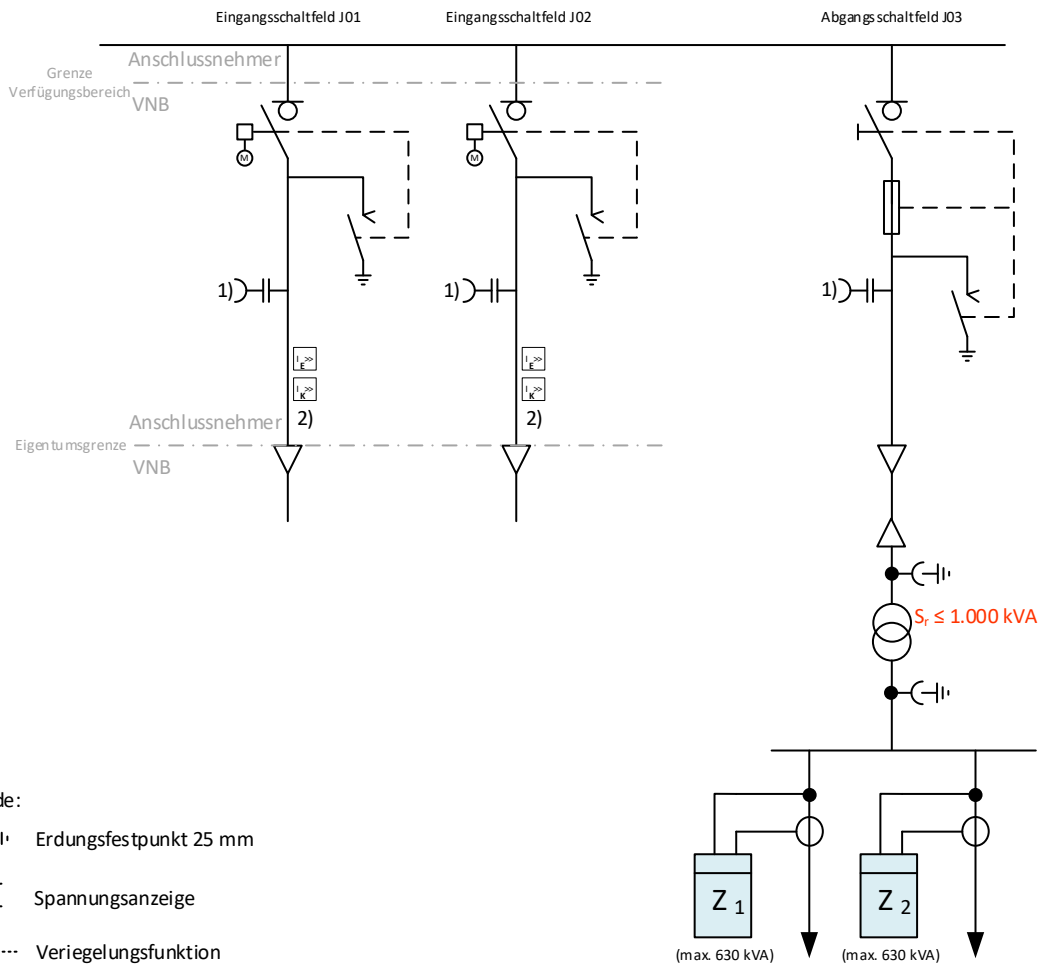
Bild 1. 20 kV-Anbindung mit einem Abgangsfeld; Transformator ≤630 kVA
